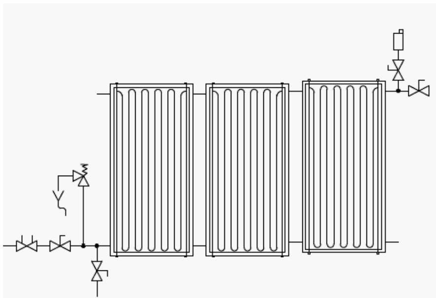
Fig. 5: Conexionado de captadores en paralelo
