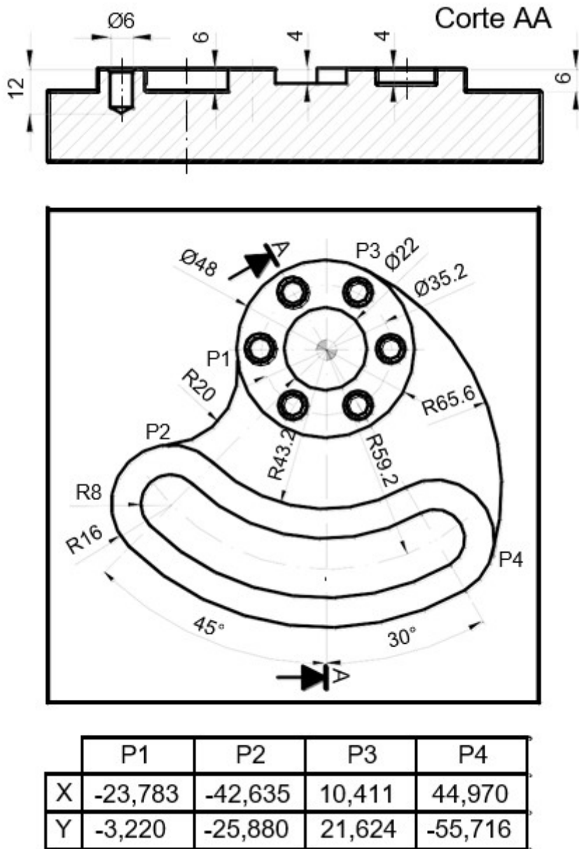
Figura 1.1. Plano de la pieza a mecanizar.
