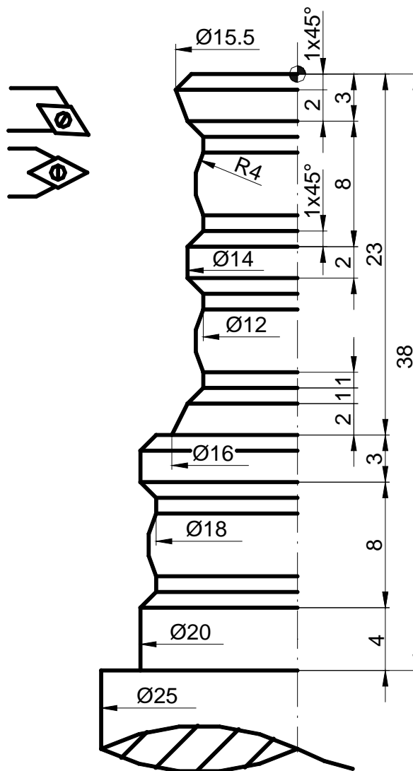
Plano de la pieza a mecanizar
